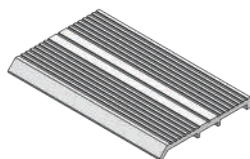
Seuil 6 mm Avec sa plinthe de 140 mm en partie basse. Double joints brosse.
