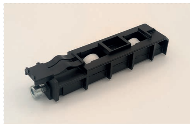
Double galets réglables à roulement aiguille, supportant jusqu'à 120 kg par vantail en standard
