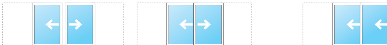
Le galandage 1 vantail sur 1 rail ou 2 vantaux sur 1 rail nécessite une épaisseur d'isolation de 180 mm
