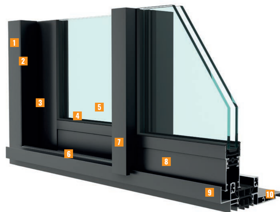
Double galets réglables à roulement aiguille, supportant jusqu'à 120 kg par vantail en standard
